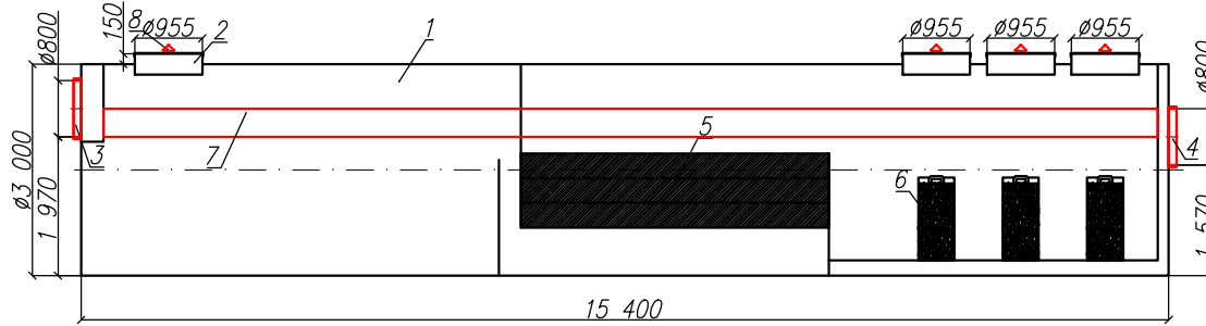
Разрез 1-1
